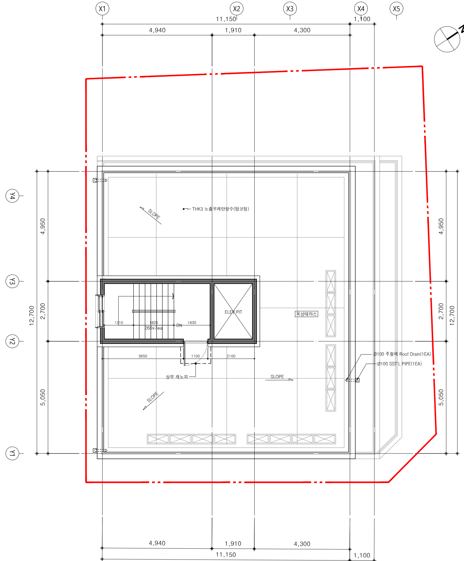
1 지붕층 평면도 SCALE : A3=1/100
