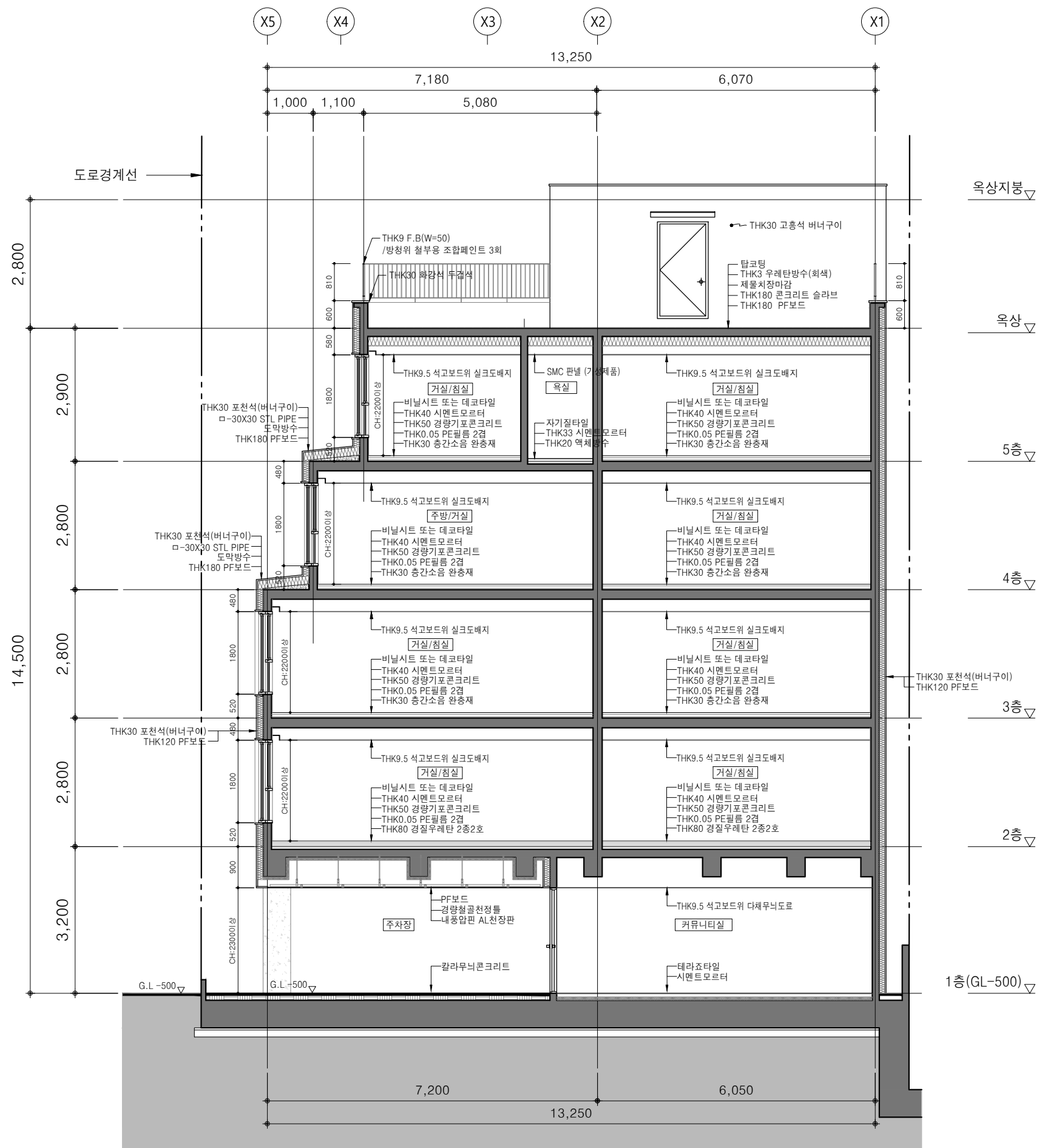
1 A 주단면도-1 SCALE : A3=1/100
