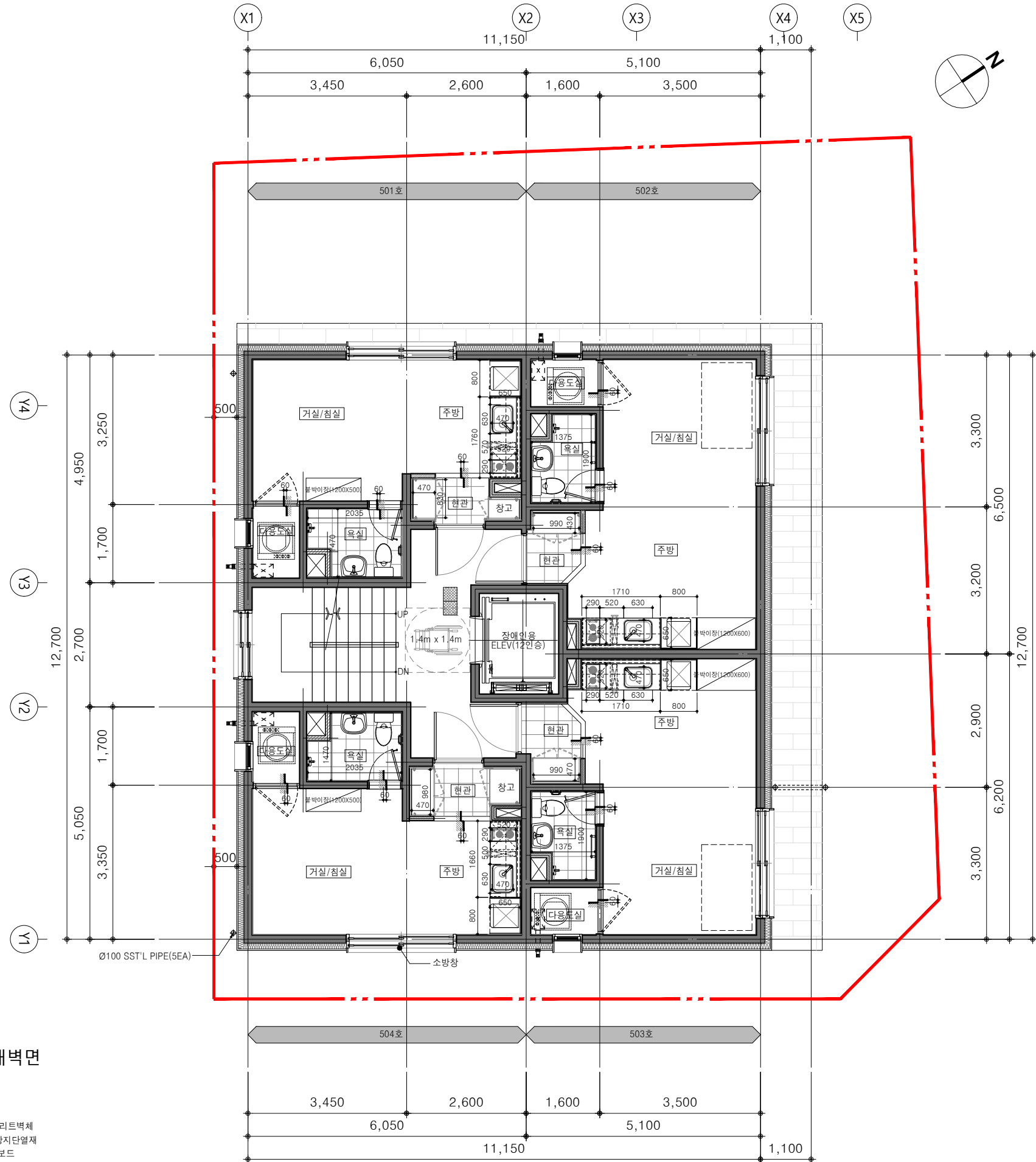
1 5층 평면도 SCALE : A3=1/100
