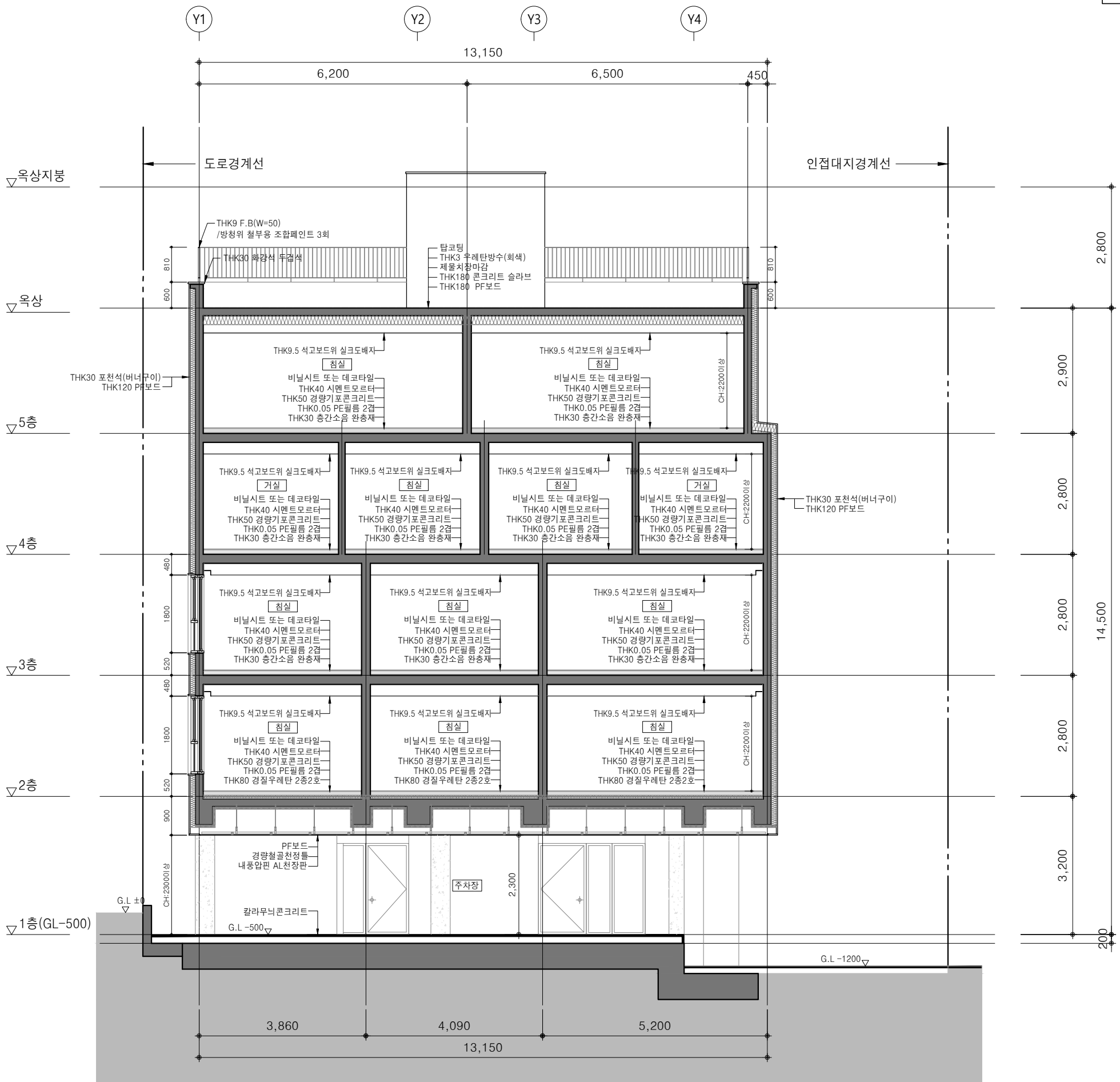
1 A 주단면도-2 SCALE : A3=1/100
