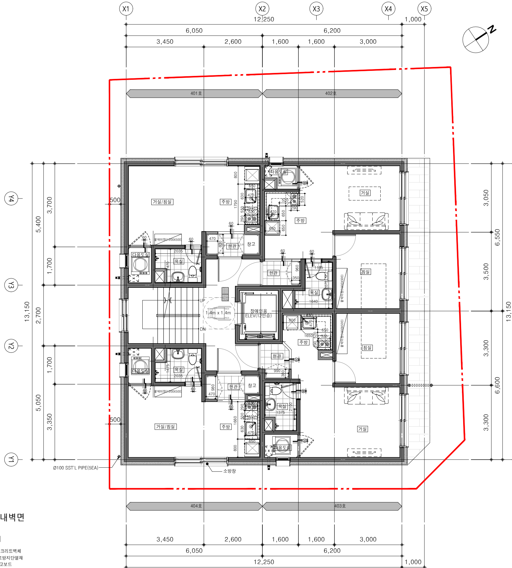
4층 평면도 SCALE : A3=1/100
