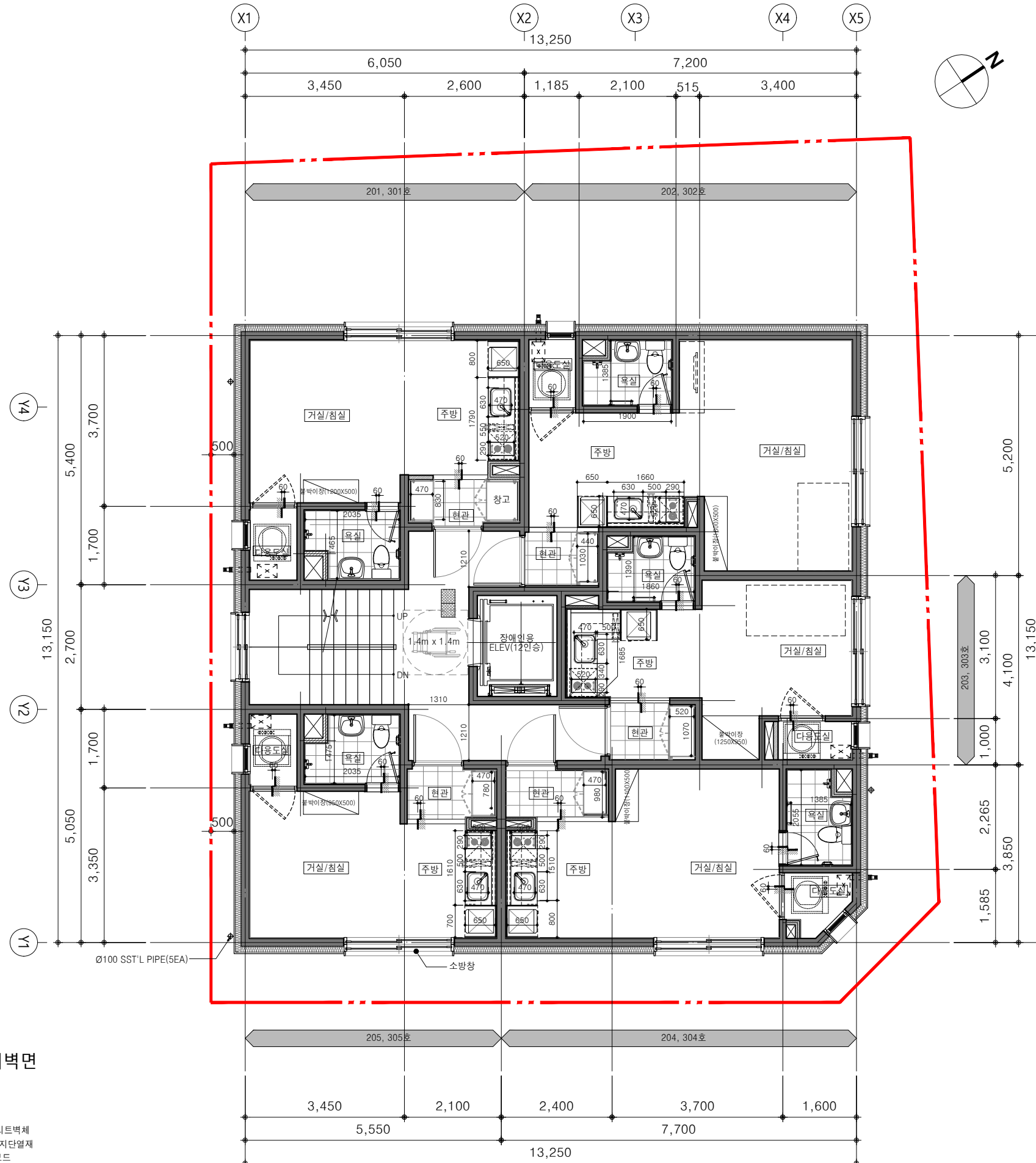
2~3층 평면도
